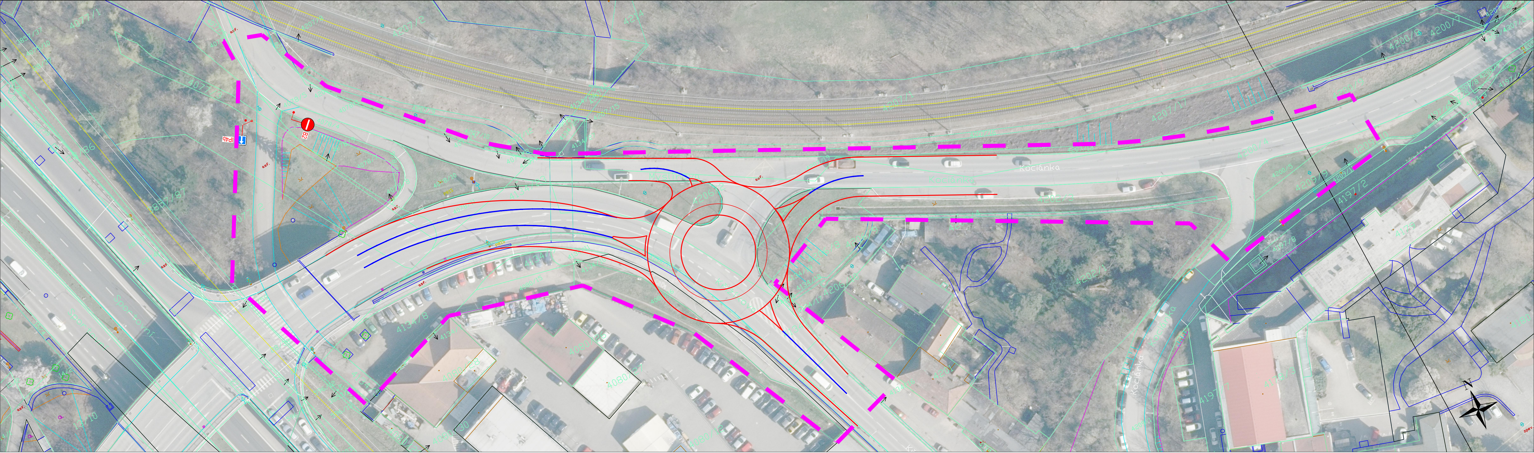
Varianta s okružní křižovatkou. Poloměr je 22 m.
